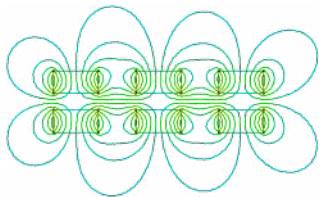
普通磁体
