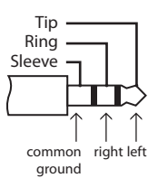
普通3.5mm立体声耳机插头
