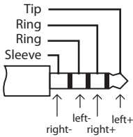
RE-600平衡插头
