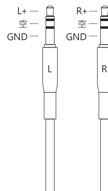
3.5mm双边耳机线 (3.5mmTRS耳机连接)
