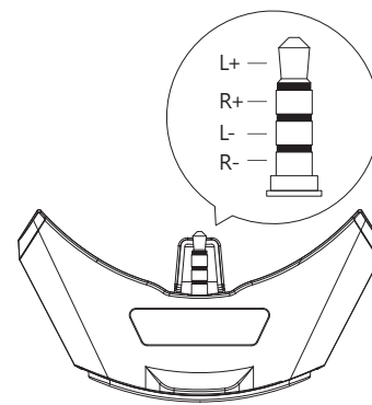
Bluemini蓝牙模块 (3.5mm TRRS耳机左侧接口连接)
